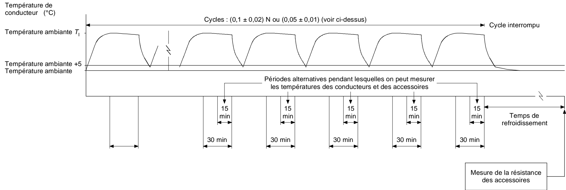
Figure D.2 - Détail de la séquence du cycle 0,1 N ou 0,05 N
